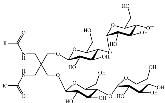
Scheme F. MNG Amphiphiles
