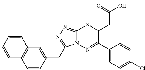
2-(6-(4-chlorophenyl)-3-(naphthalen-2-ylmethyl)-7H-[1,2,4]triazolo[3,4-b][1,3,4]thiadiazin-7-yl)acetic acid (4.5.17)
