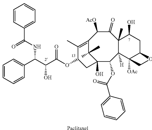
Paclitaxel
